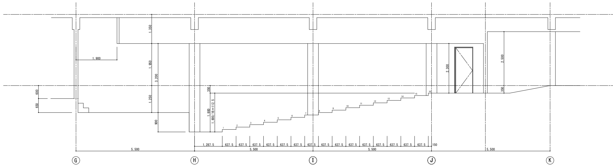
通路部分断面图
